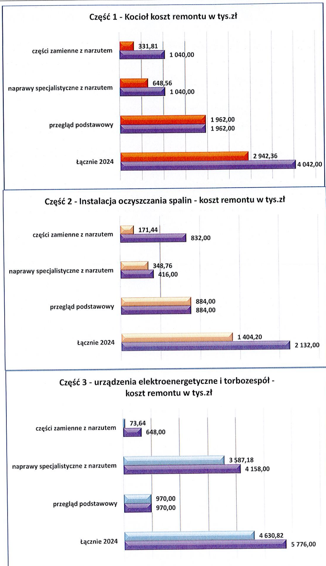
Wykres 24 Źródło: opracowanie własne MZGOK Sp. z o.o. na podstawie prowadzonych ewidencji
